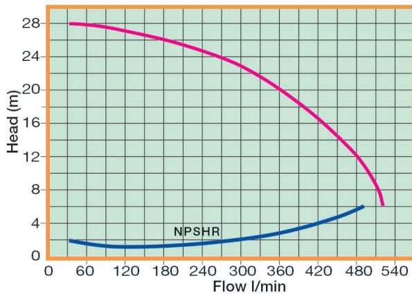
Curva caratteristica 50 Hz
