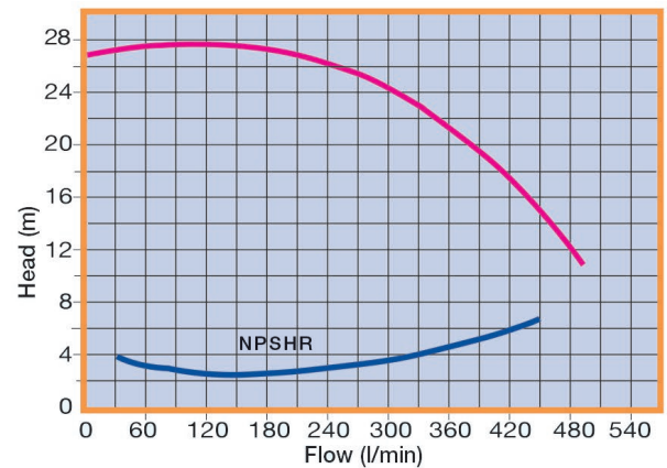
Curva caratteristica 60 Hz
