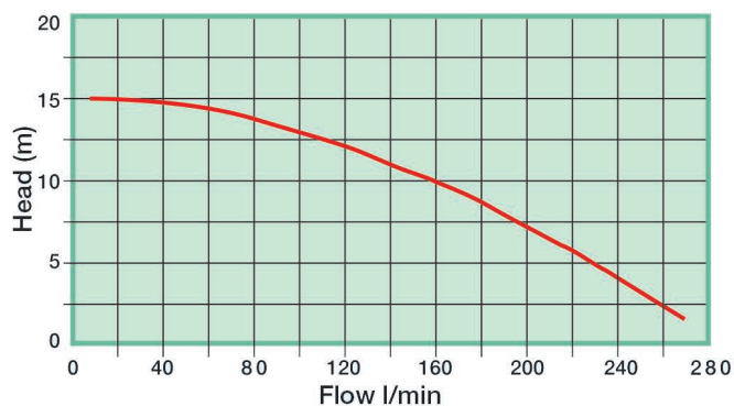
Curva caratteristica 50 Hz - Rpm 2800
