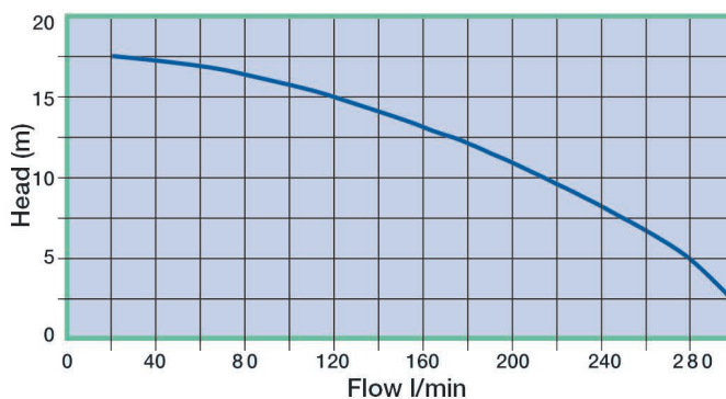
Curva caratteristica 60 Hz - Rpm 3400
